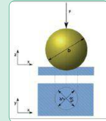
5.56-3 Essai Vickers
