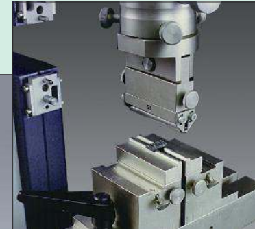
5.52-3 Appareil de test de cisaillement
