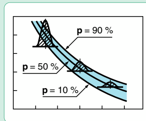
5.54-5 Courbes de probabilité de rupture
