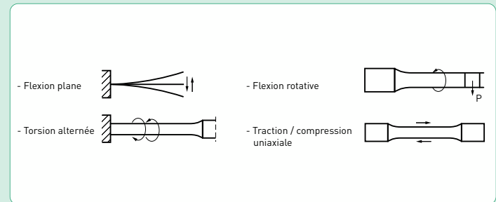
5.54-2 Types de sollicitation pour essais de fatigue
