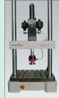
5.54-7 Machine de test uni-axiale
