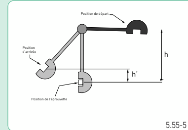
5.55-5 Représentation du mouton-pendule et des hauteurs à prendre en compte pour le calcul de l'énergie absorbée
