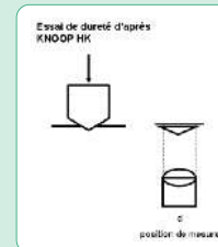
5.56-4 Essai Knoop
