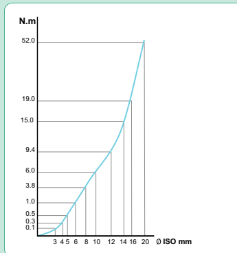
5.4-2 Courbe de résistance à la traction PA 6-6
