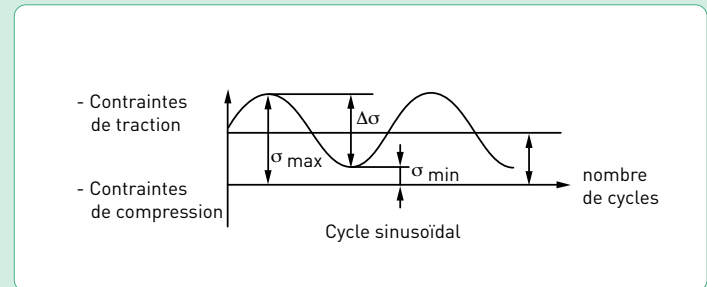
5.54-3 Exemple de courbe d'essai de fatigue
