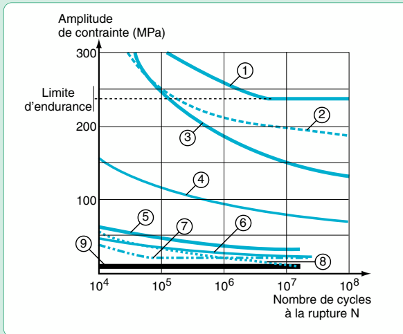
5.54-4 Courbes de Wöhler
