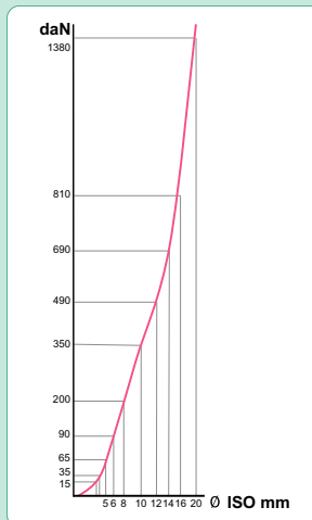
5.4-2 Courbe de résistance à la traction PA 6-6
