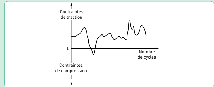
5.54-1 Exemple de courbe de fatigue en situation réelle
