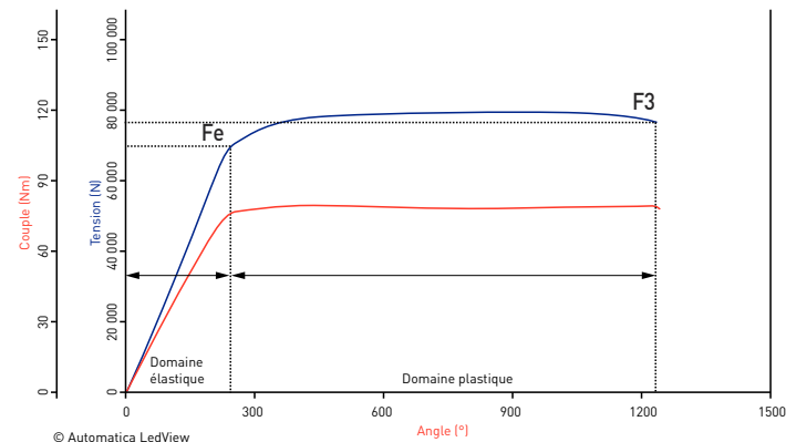
5.57-3 Exemple de courbe de serrage dans le domaine plastique
