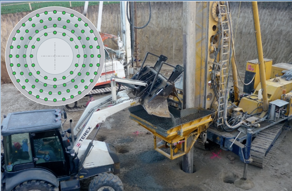
Vibro Concrete Columns
