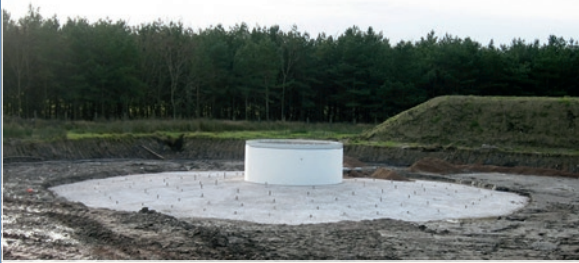
Vibro Stone Columns
