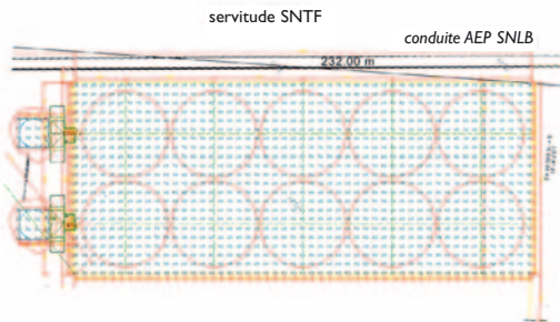
▲ Plan d'implantation des colonnes ballastées
