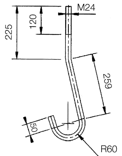
Tige d'ancrage \varnothing 24
