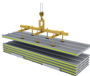
Manutention par palonnier à ventouses
