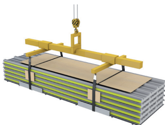
Manutention par élingues plates
