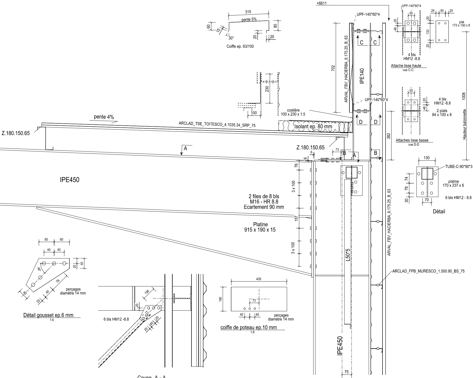
Élévation 1:8
