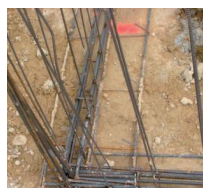
Noeud de chaînage - Continuité mécanique
